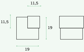
IN.13.119.P QUADRO Material: EN 1.4301 - Polido / Polished / Pulido Batente de chão / Door stopper / Tope de puerta.
